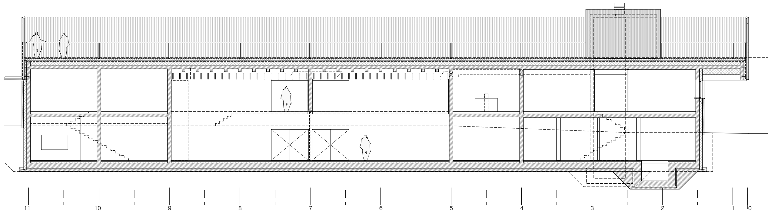
Schnitt A-A
