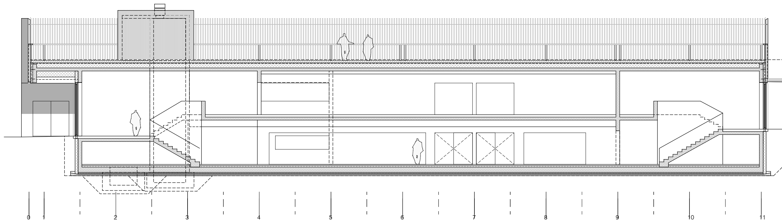
Schnitt B-B
